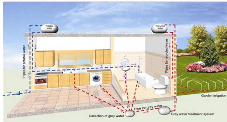
Figure 10 – Système de réutilisation des eaux grises à Chypre Source : EC Europa
