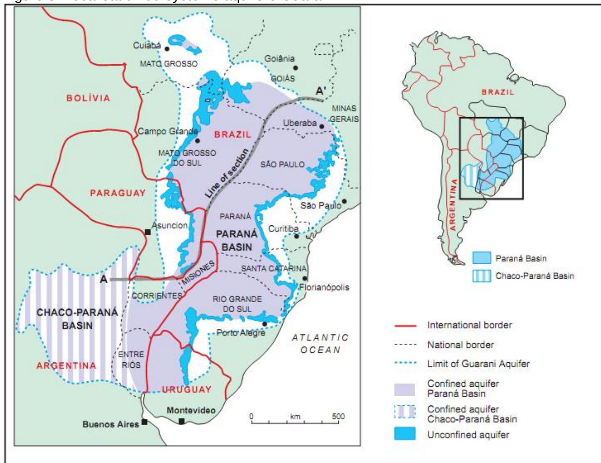
Figure 3: Localisation du système aquifère Guaraní e .
