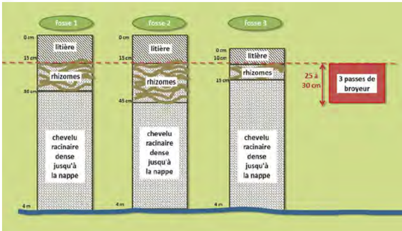
Comparaison entre la capacité de pénétration de l'engin dans le sol et la profondeur des rhizomes.
