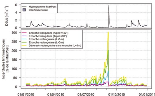
Figure 4 : Incertitudes limnimétriques des débits moyens horaires sur l'année 2010, au cours du temps (à gauche) et en fonction des débits classés (à droite) pour les cinq configurations de stations hydrométriques fictives. Les incertitudes relatives sont exprimées en pourcentage du débit issu de la courbe de tarage calculée par BaRatin (« MaxPost »).
