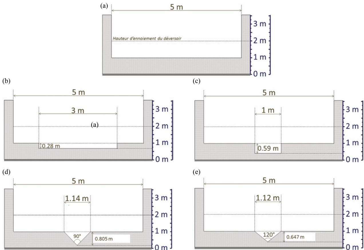
Figure 1 : Caractéristiques géométriques des déversoirs des cinq stations hydrométriques fictives étudiées : seuil rectangulaire initial (a), avec encoche rectangulaire de 3 m (b) ou de 1 m (c), avec encoche triangulaire de 90° (d) ou de 120° (e).
