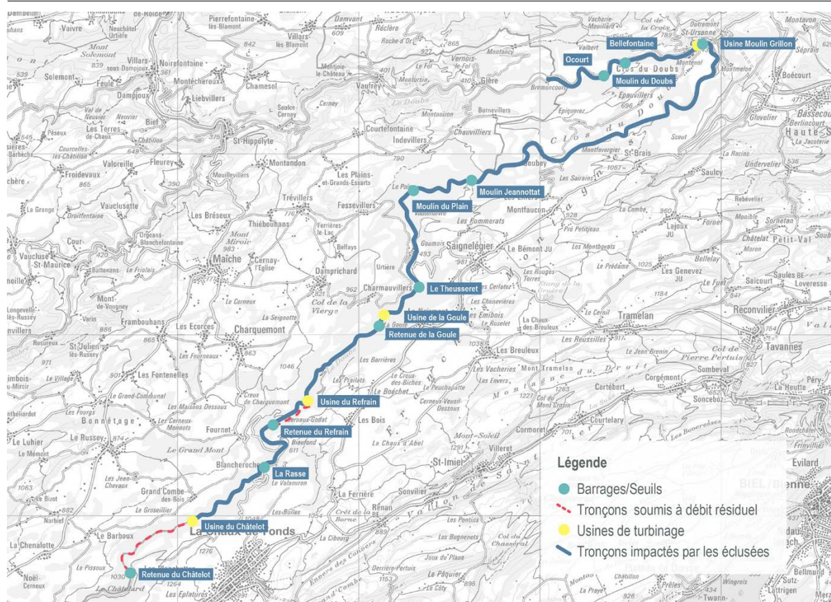
Fig. 9 Localisation des principaux ouvrages hydroélectriques et seuils sur le Doubs frontière et jurassien
