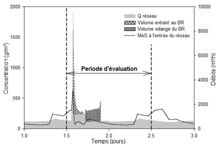
Figure 4 : Intrants correspondant à chaque bassin versant. La première journée, servant à définir les conditions initiales, n'est pas représentée. En gris, le débit généré par le bassin versant et en tacheté, le débit de vidange du bassin de rétention (BR) pour le scénario de référence. En trait plein, la concentration en MeS à l'entrée du réseau.
