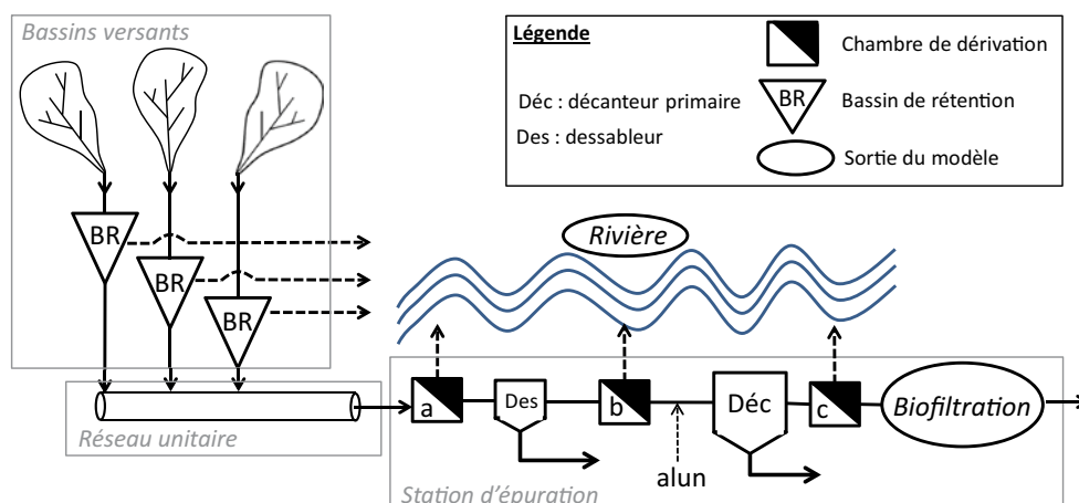
Figure 1 : Schéma de la configuration du système intégré comprenant les bassins versants, la STEP (dessableur, décanteur primaire et biofiltration) et le milieu récepteur.
