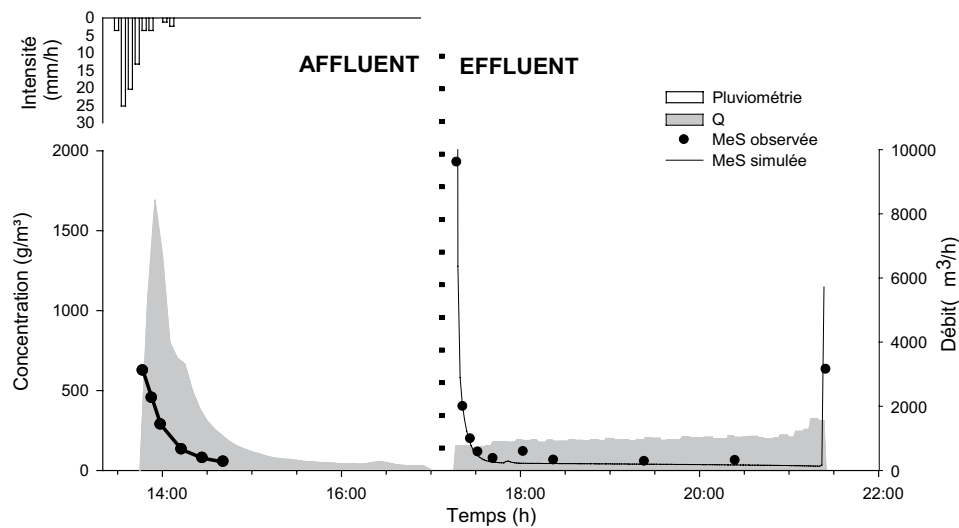
Figure 2 : À gauche, pluviogramme et caractéristiques de l'affluent du bassin de rétention de Saint-Sacrement (remplissage). À droite, caractéristiques de l'effluent du bassin de Saint-Sacrement (vidange). En vidange, le trait plein correspond aux MeS simulés [Maruéjols et al. (2013b)]. Évènement du 27 juillet 2009 à Québec, Canada.
