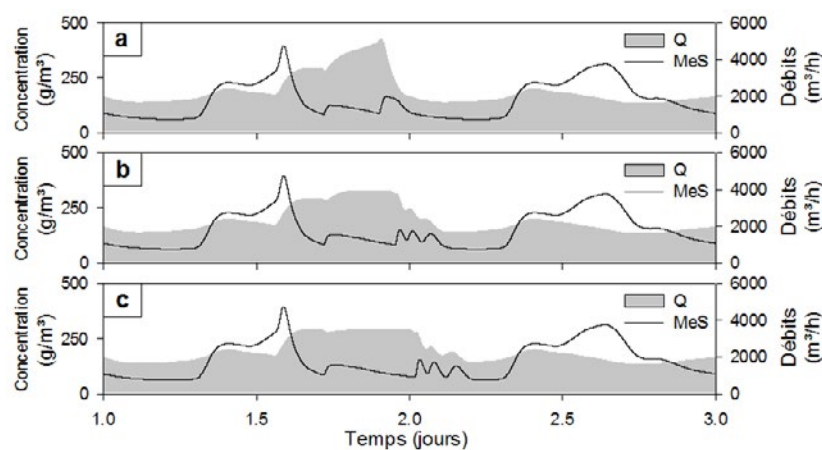
Figure 5 : Débits et MeS arrivant à la STEP : (a) pour les scénarios 0, 1 et 2; (b) pour les scénarios 3, 4 et 5; (c) pour les scénarios 6, 7 et 8.
