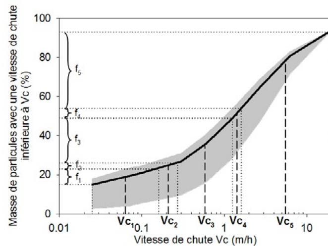
Figure 3 : Zone typique de DVCP observée dans le réseau (en gris). Un exemple de fractionnement de la MeS en cinq classes de particules est illustré. Chaque classe de particules, caractérisée par une vitesse de chute moyenne ( V_{c1} à V_{c5} ), est associée à sa fraction massique de MeS ( f_1 à f_5 ), donnée par les accolades.
