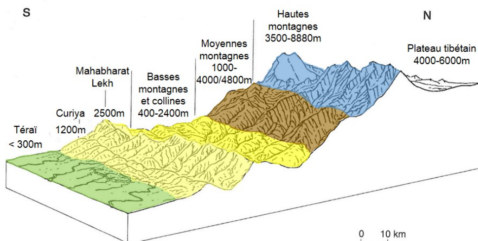
Figure 2. Bloc diagramme nord-sud de l'Himalaya népalais
