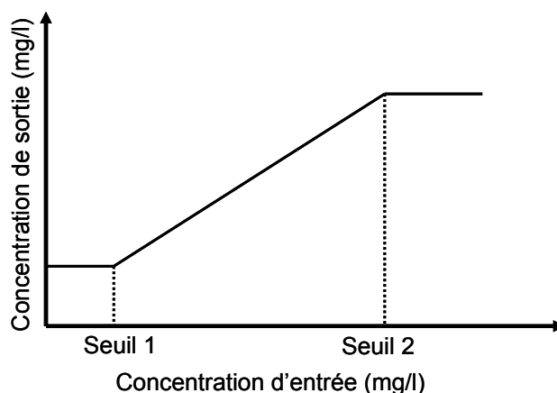
FIGURE 7 : RELATION ENTRE CONCENTRATIONS D'ENTRÉE ET DE SORTIE
