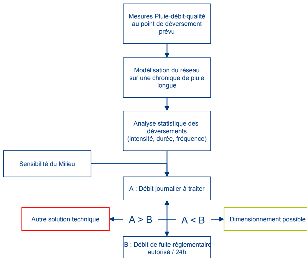
FIGURE 16 : SYNOPTIQUE DE LA DÉMARCHE POUR DÉTERMINER LA FAISABILITÉ TECHNIQUE D'UN OUVRAGE DE FPR
