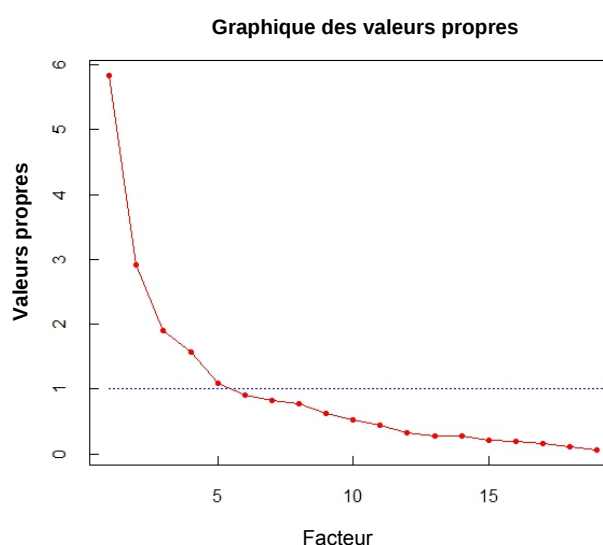
Figure 14 : Graphique des valeurs propres montrant les valeurs propres initiales et les facteurs obtenus à partir de l'ACP.
