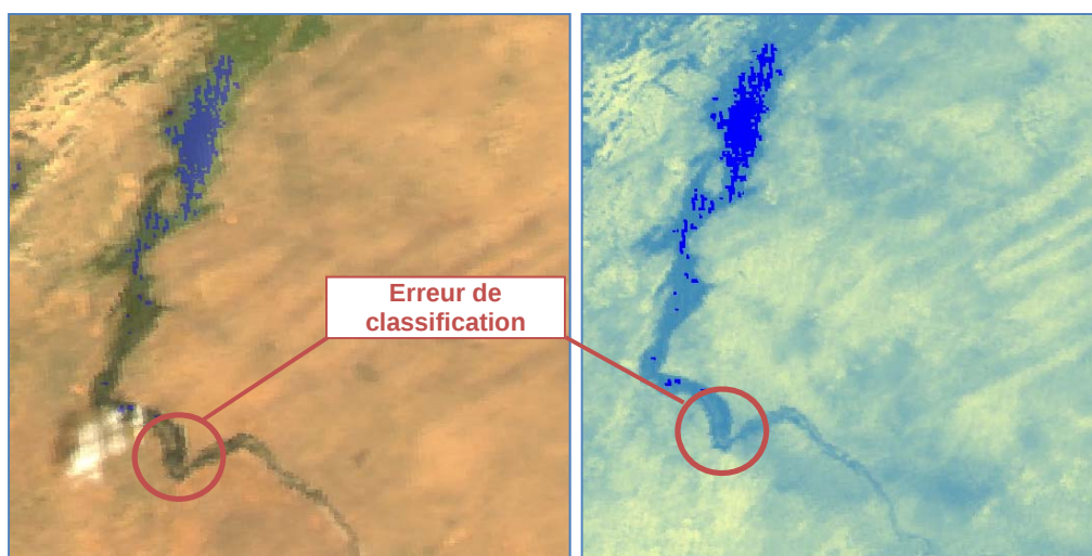
Figure 1 : Les zones de détection de l'eau où les valeurs de seuil standard de l'algorithme de classification de DFO ont classé de manière erronée des étendues d'eau comme étant des sols. (À gauche : le lac de Guiers dans le spectre visible ; à droite : le lac de Guiers en infrarouge proche PIR – SWIR en anglais).
