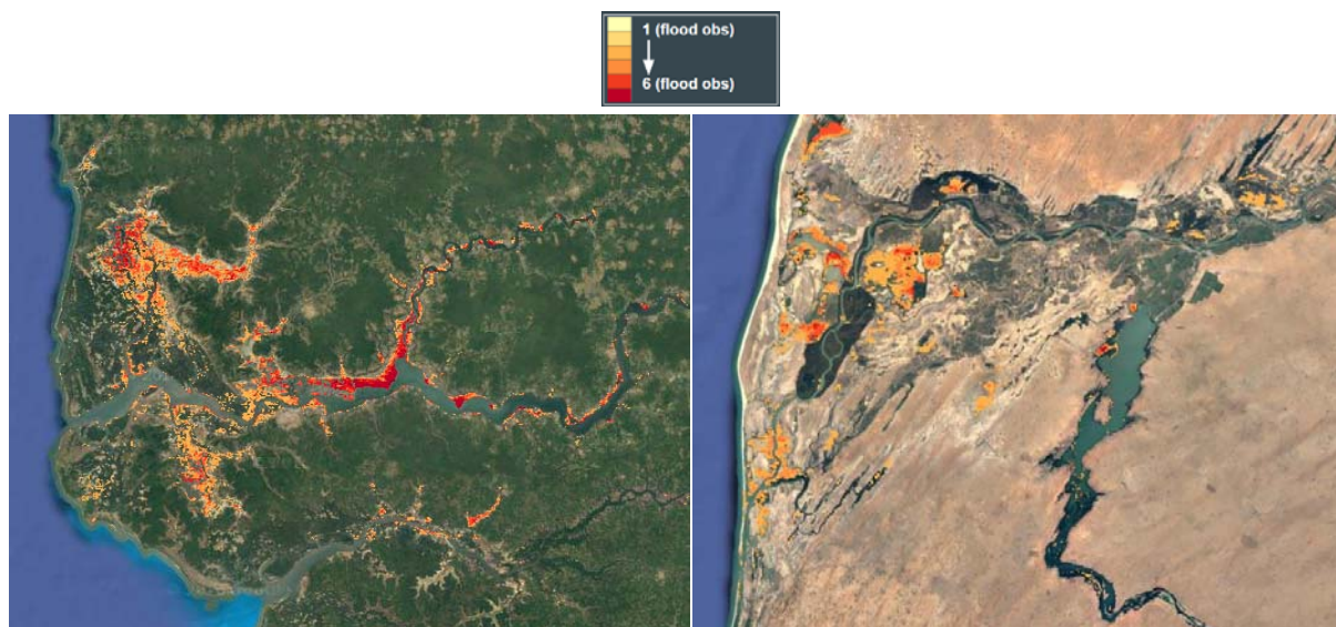
Figure 2 : Nombre de fois qu'une zone (pixel) a été inondée entre 2003 et 2015 au Sénégal en utilisant l'algorithme de DFO (à gauche : Ziguinchor, Sénégal ; à droite : Saint-Louis, Sénégal et fleuve Sénégal).
