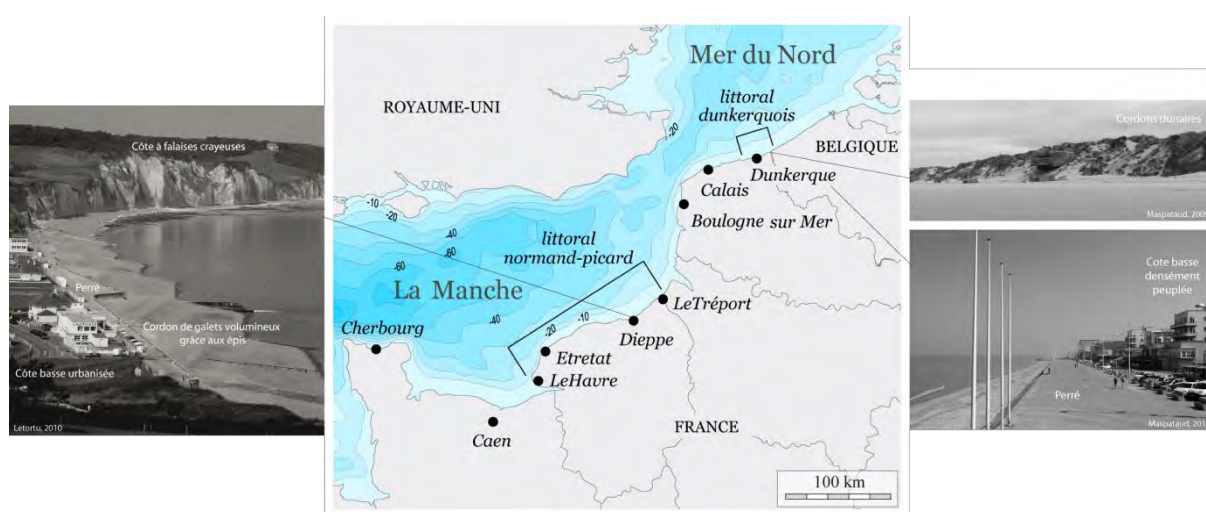
Figure 1 : Localisation des secteurs d'étude en Manche orientale et Mer du Nord méridionale.
