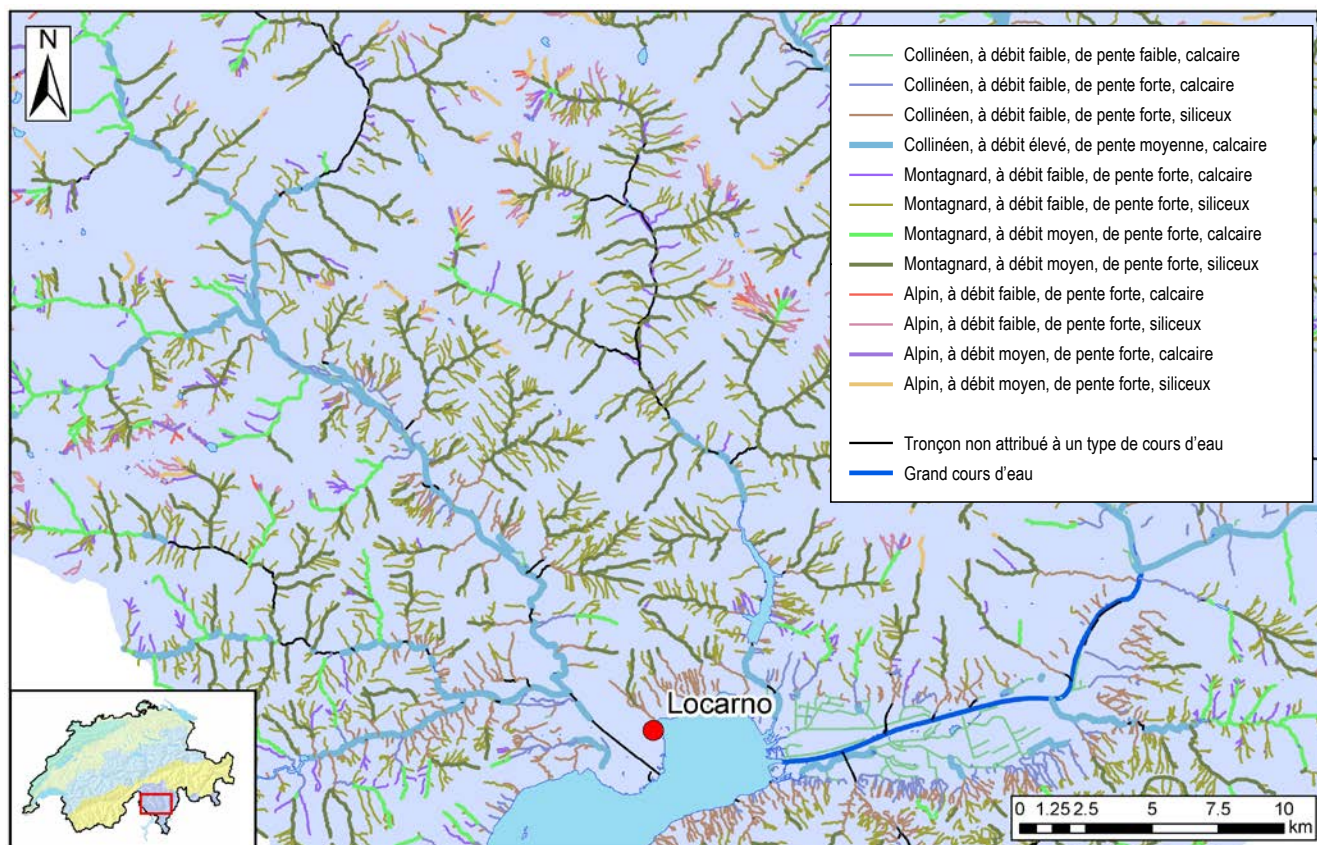
Fig. 7 &gt; Typologie des cours d'eau dans la région biogéographique Versant sud des Alpes
