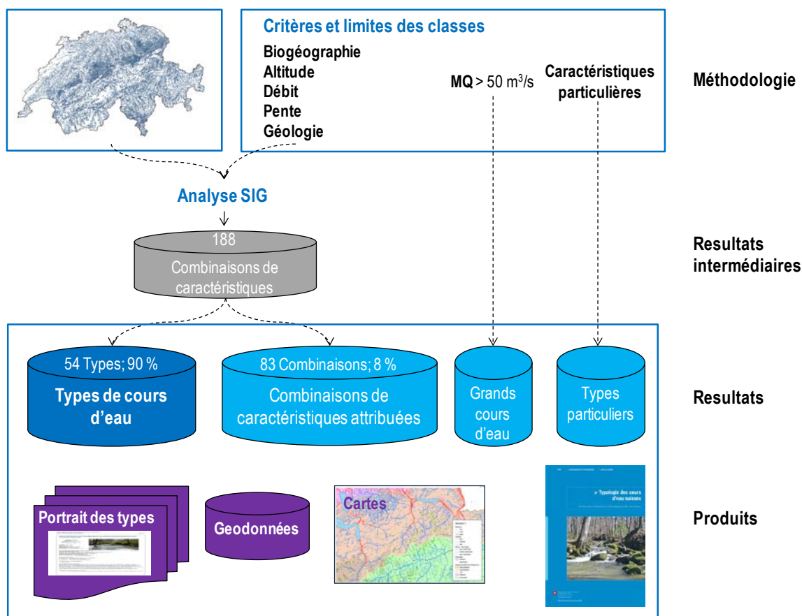
Fig. 1 > Méthode appliquée, résultats et produits de la typologie des cours d'eau
