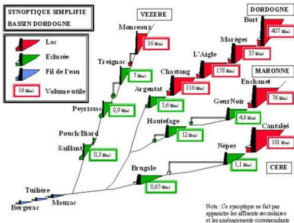
Figure n°10 : Synoptique simplifié du bassin versant de la Dordogne (p.17 de l'Etude du schéma de cohérence entre la production d'hydroélectricité et le bon état des milieux aquatiques sur le bassin versant de la Dordogne, rapport, 2012)
