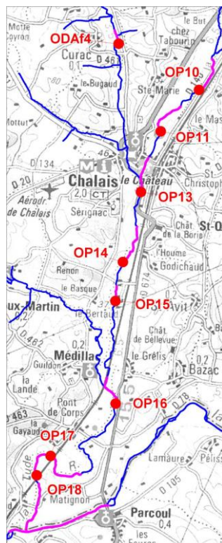
Figure n°35 : Situation spatiale des 9 ouvrages concernés par la CECE (source : étude pour la restauration hydromorphologique et la continuité écologique de la Tude, de la Dronne charentaise, de leurs affluents et astiers, GEODIAG, 2015)
