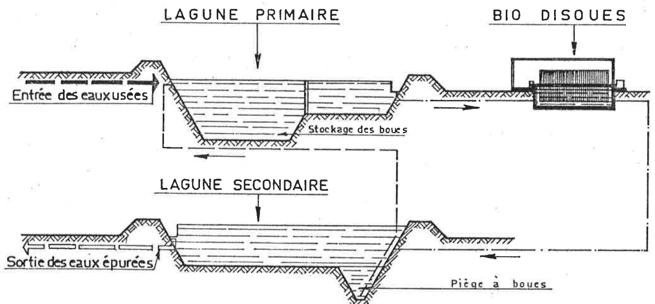
Schéma de principe - Vue en coupe.
