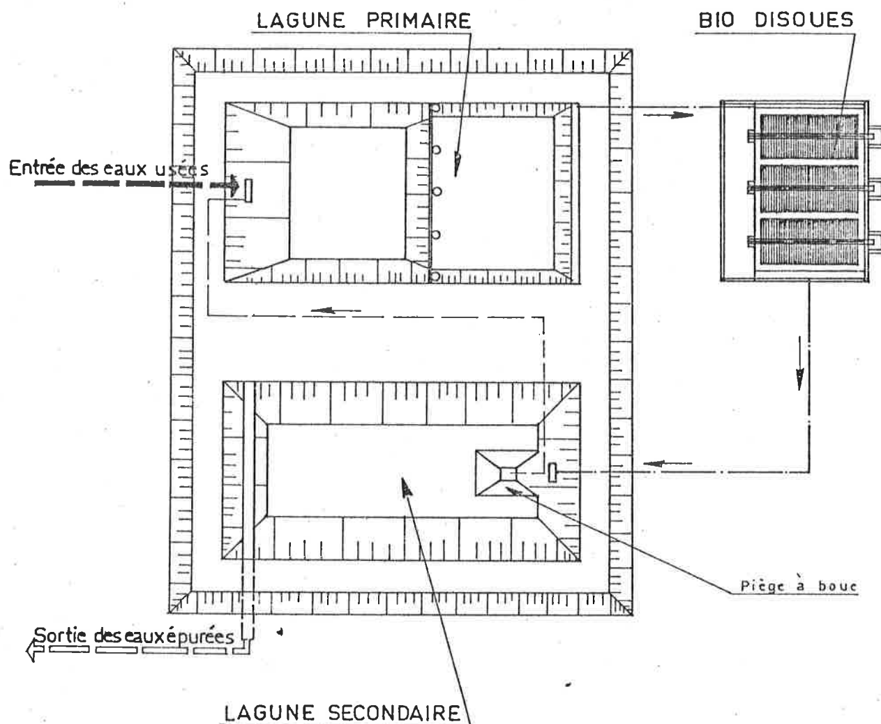
Schéma de principe - Vue en plan.
