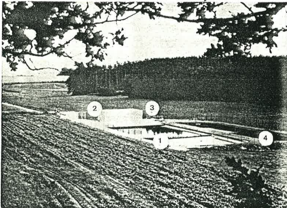
Vue d'ensemble d'une installation de lagune activée par BIO-DISQUES.
