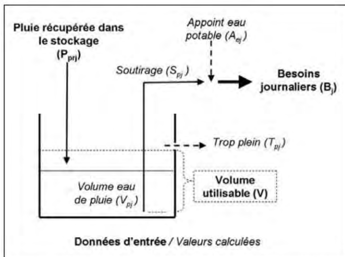
Figure 4. Flux d'un système de récupération et d'utilisation d'eau de pluie
