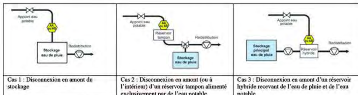
Figure 11. Localisations possibles du dispositif de disconnexion
