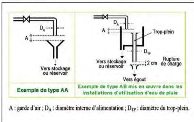
Figure 14. Exemples de disconnexions de types AA et AB
