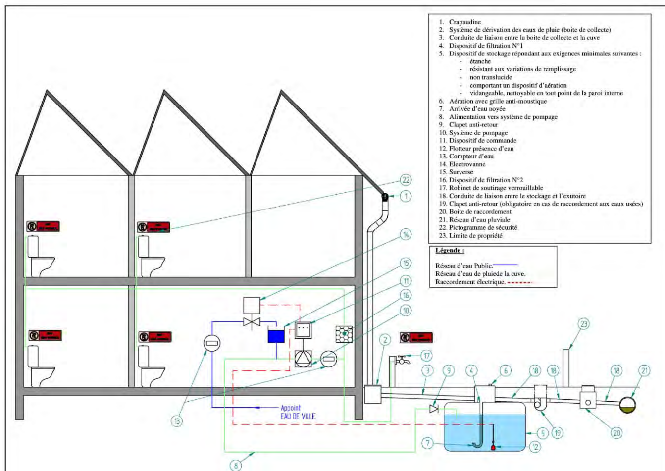
Figure 10. Installation pour bâtiment industriel avec usage intérieur et trop-plein relié au réseau
