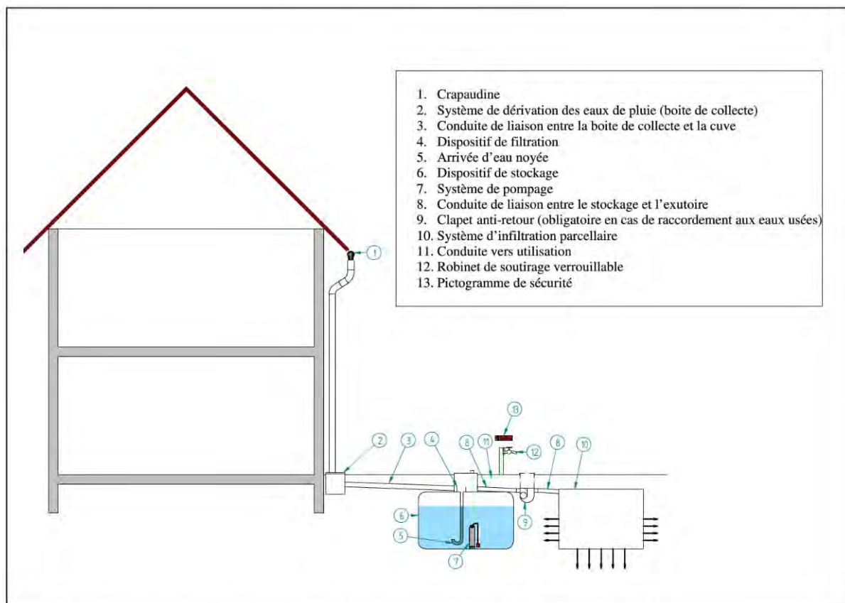
Figure 6. Installation enterrée à l'extérieur du bâtiment avec usage extérieur et infiltration du trop-plein
