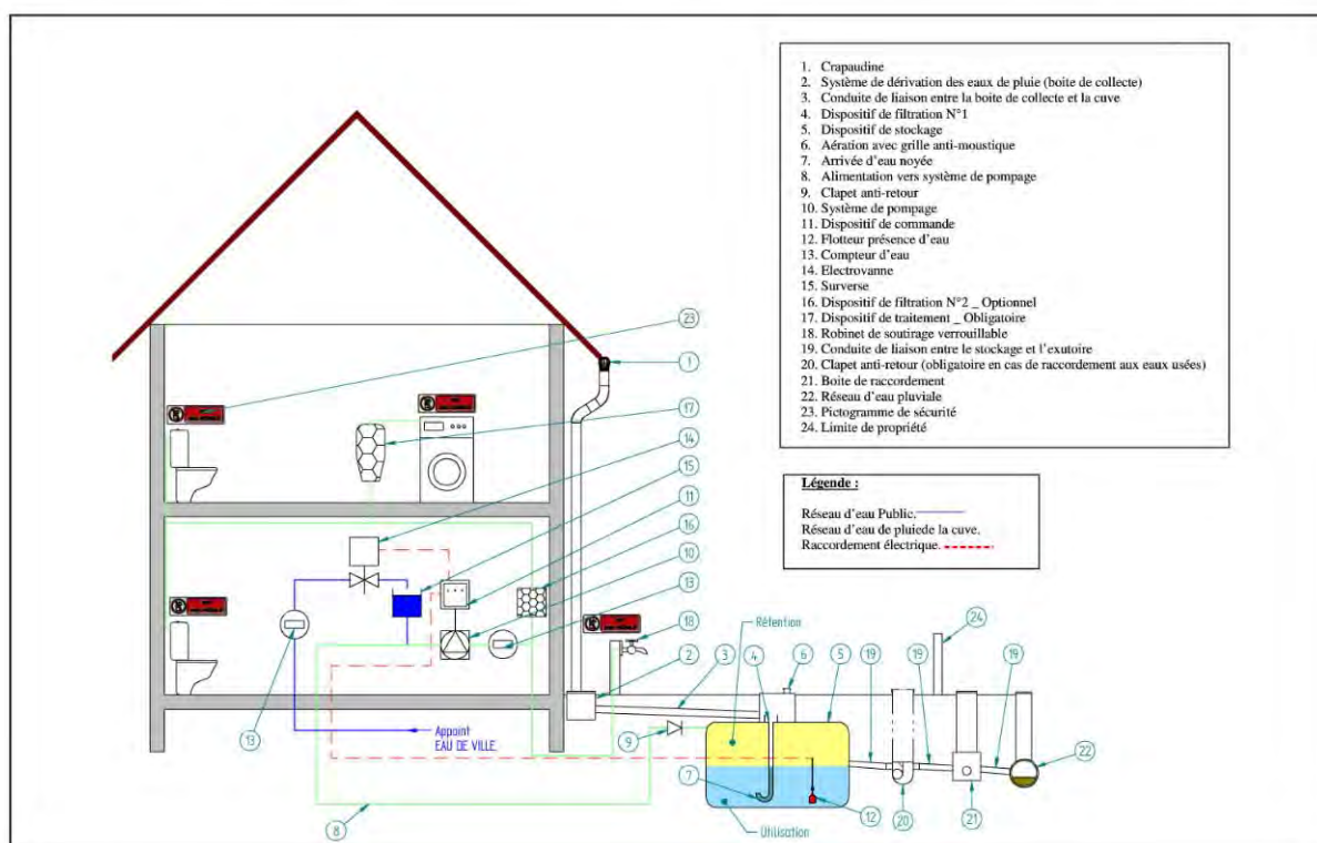
Figure 7. Installation avec stockage en sous-sol du bâtiment avec usages intérieur et extérieur et trop-plein rejetant au réseau
