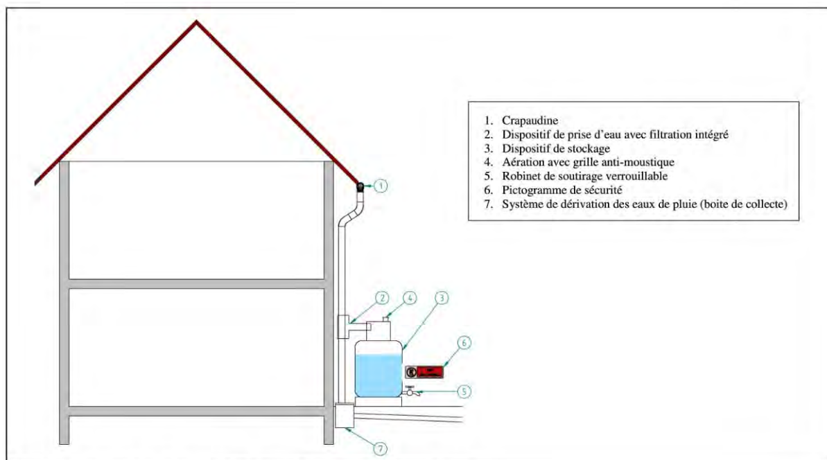
Figure 9. Installation avec stockage non enterré et usages extérieurs seuls
